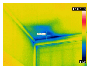
雨漏り箇所の温度が低い(青)
