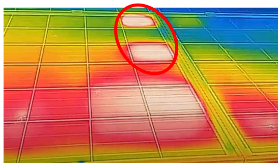
太陽電池の異常部の温度が高い(白)
